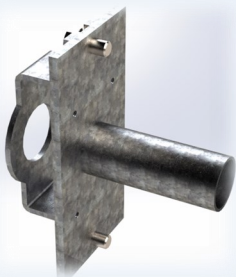
Porte Verrou : Taroudage M5 - 75 x 49
